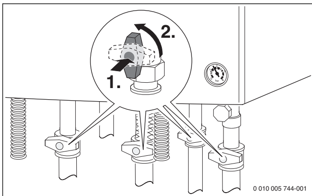
Фиг. 2 Отваряне на сервизните кранове
